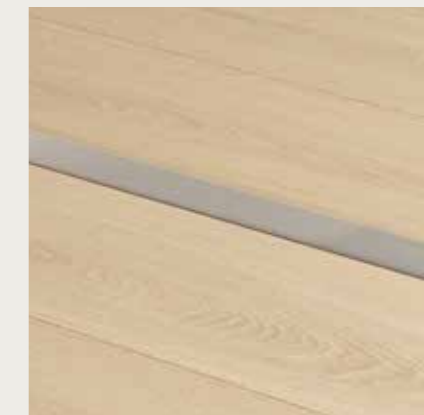
PROFILO DI ESPANSIONE 2000 x 34 x 7 mm Per coprire lo spazio di dilatazione tra due pavimenti della stessa altezza. Materiale: alluminio. SFEXPSILV | SFEXPCOFF | SFEXPCLAY | SFEXPCHAM | SFEXPBLACK
